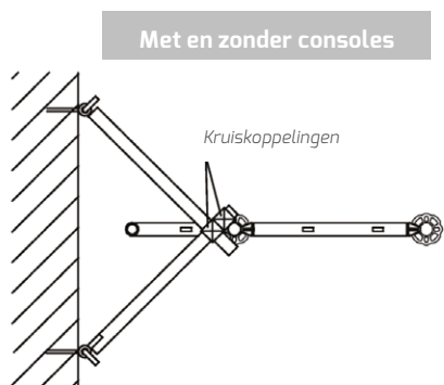
FIGUUR 22: V-verankering
