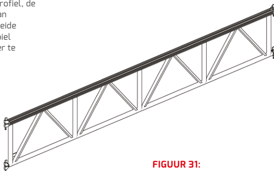
FIGUUR 31: U-Tralieligger
